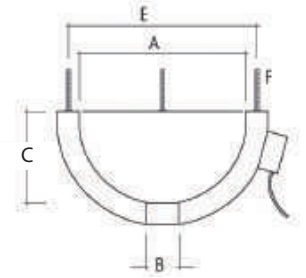
Schematischer Aufbau einer Industrieheizhaube
